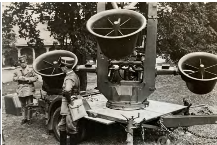
Fig. 6 a & b. Lyssnarapparat VD3 m/36 i olika positioner.
