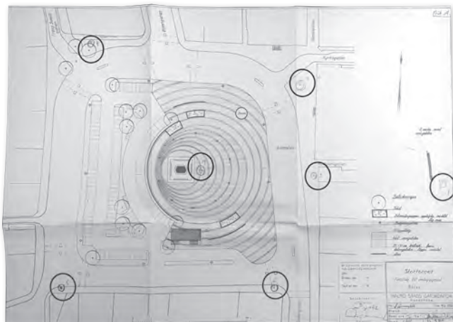
Fig. 8. Mätstationerna för den första mätningen av ljudnivån från det planerade klockspelet på Kompanigården. Ringarna markerar mätstationerna och är ditsatta av författaren för att markera mätstationerna på ritningen.
