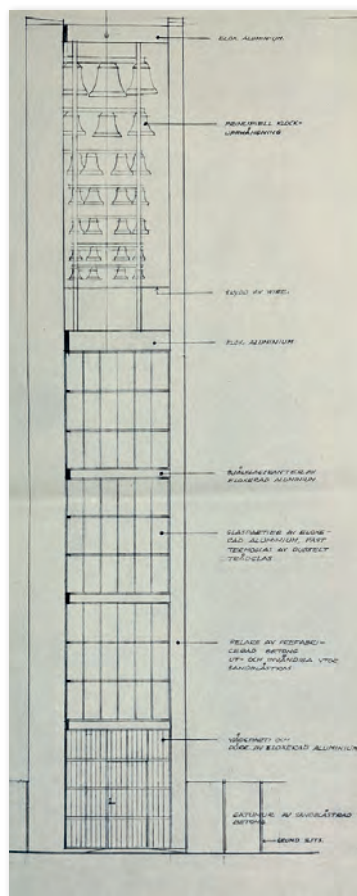
Fig. 13. Det slutliga förslaget till utformning av klocktornet, med helt nytt utseende med natureloxiderad aluminium och trådarmerat fönsterglas. Bygglov beviljat den 6 maj 1969.
