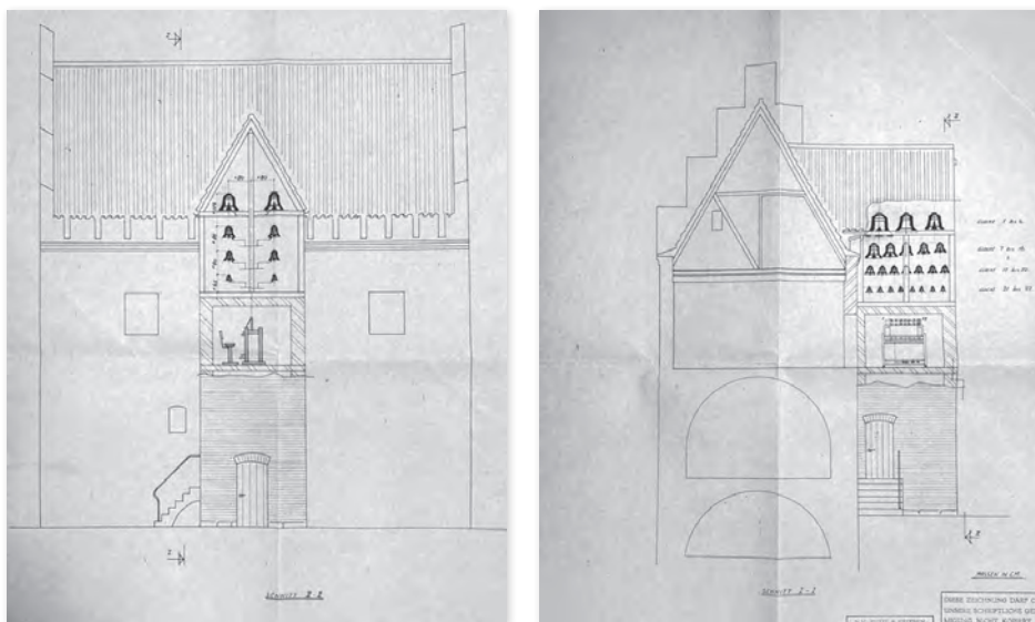
Fig. 9 A och B. Ritningar på Kompanihuset med klockspel med 47 klockor i trapphustornet, utförd av N.V. Petit & Fritsen, Nederländerna, 19 januari 1967.
